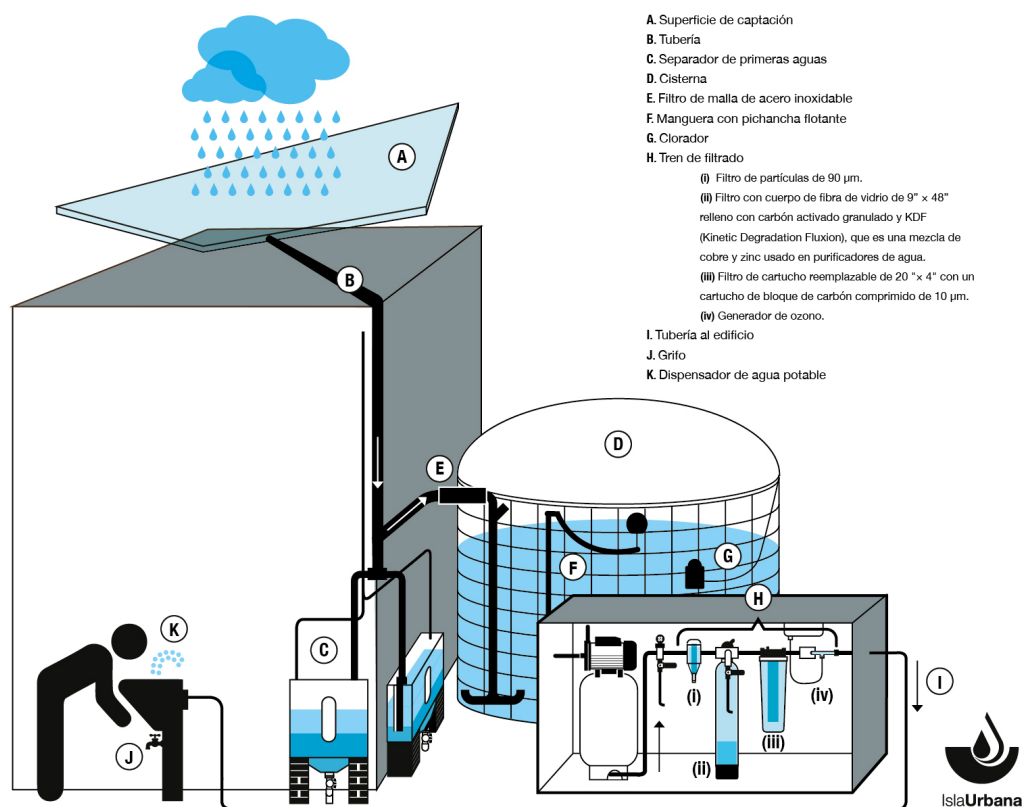
Figura 1. Diagrama del sistema de captación de agua de lluvia.
