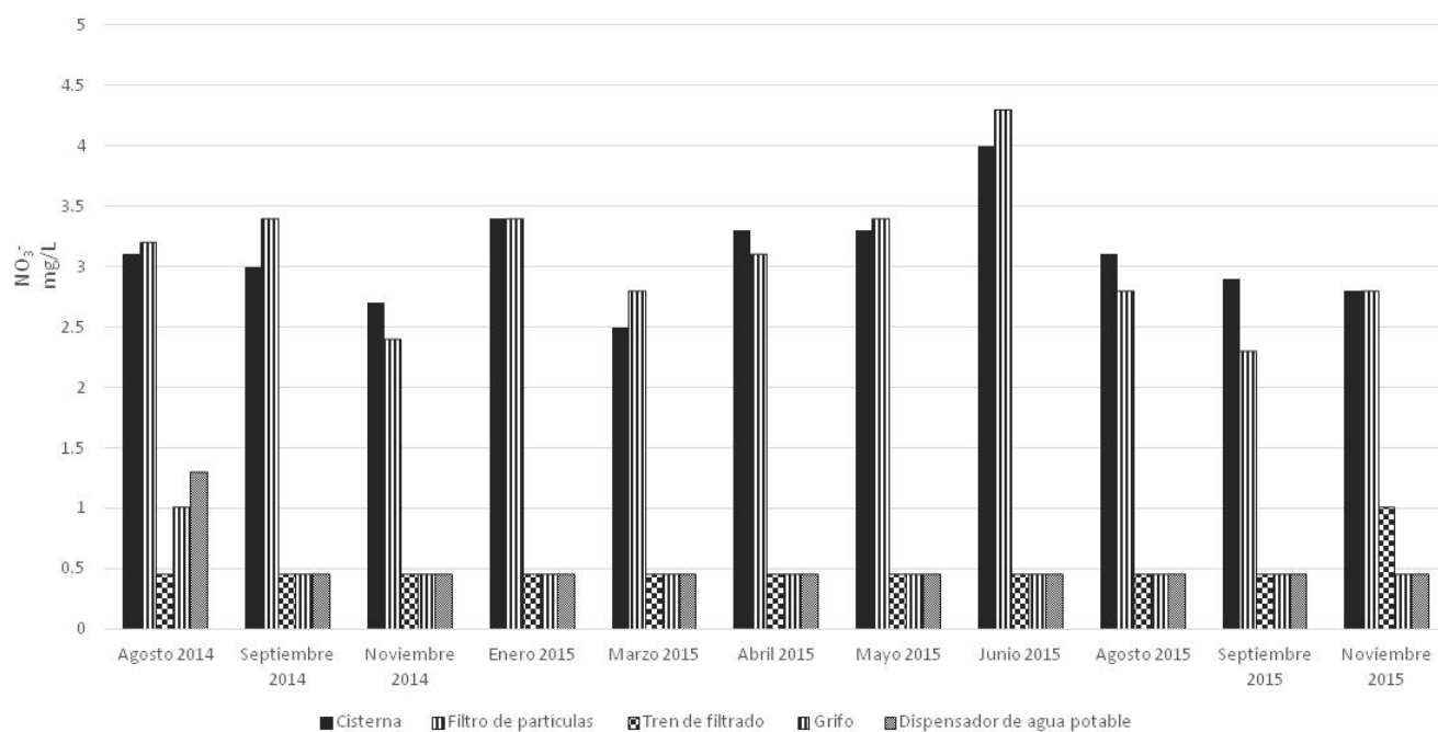
Figura 2. Concentración de nitratos en el sistema de captación de agua de lluvia durante el periodo de muestreo.
